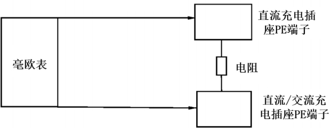
图5 电位均衡（可导电部件间）检测示意图
