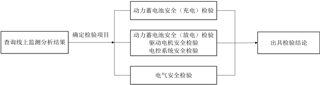
图1 新能源汽车运行安全性能检验流程
